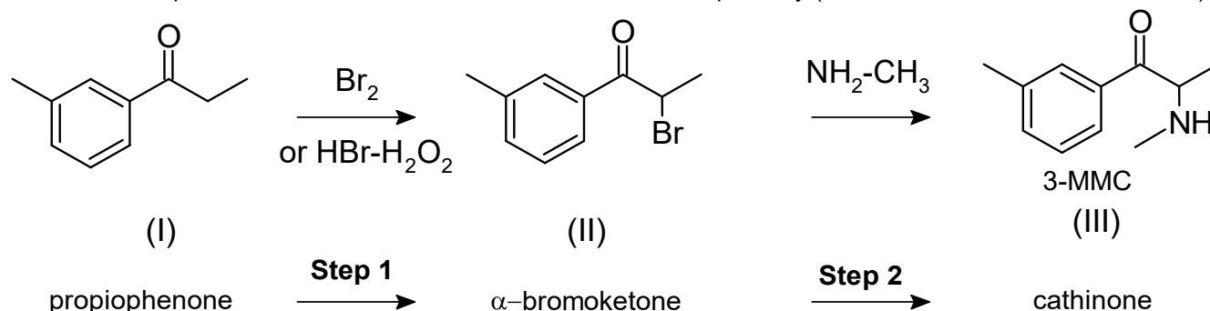
Scheme 1. Preparation of 3-MMC via the 'bromination-amination' pathway (Power et al., 2011; Wrzesień, 2018).
